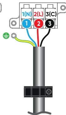
Bornier unité intérieure B
