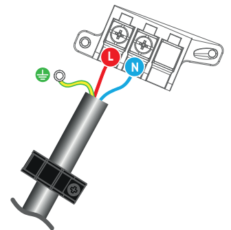
Alimentation de l'unité extérieure
