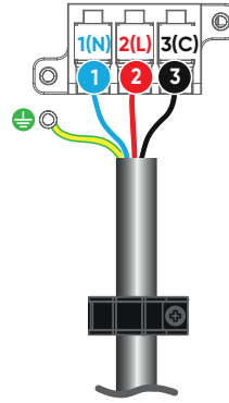
Bornier unité intérieure D
