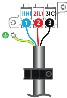
Bornier unité intérieure B
