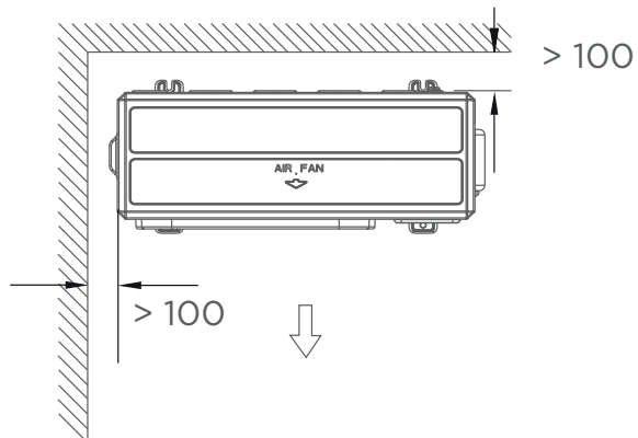
Obstacles derrière et sur un côté
