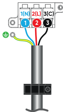
Bornier unité intérieure C
