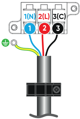
Bornier unité intérieure A
