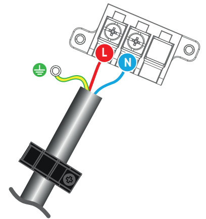
Alimentation de l'unité extérieure
