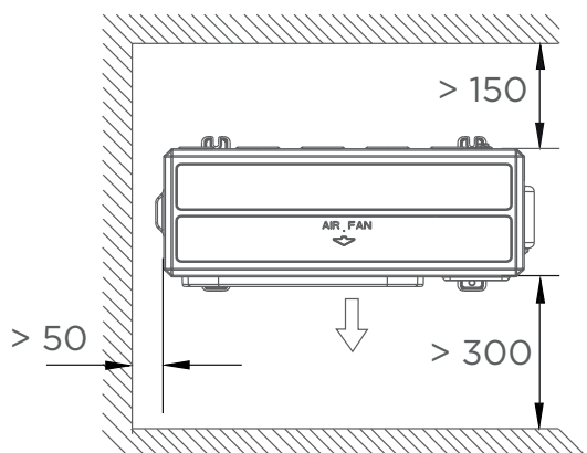
Obstacles devant, derrière, côté
