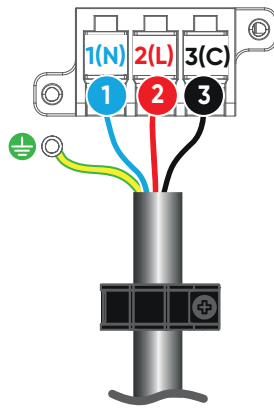
Bornier unité intérieure C
